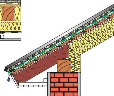
a) átszellőztetés nélkül
