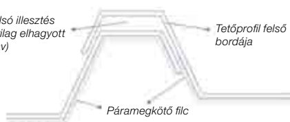
3. ábra: A kapilláris vízfelszívódást meg kell akadályozni az illesztéseknél és az eresztűlnyúlásnál
