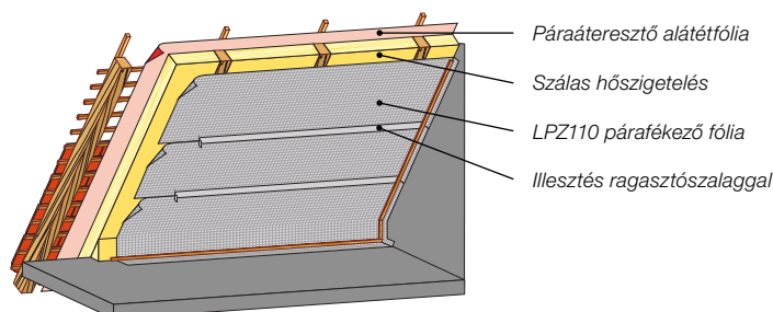
Beépített tetőtér, hőszigetelt fa tetőszervezet
