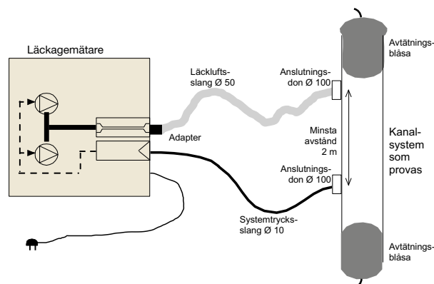
Bild 2: Mätprincip, täthetstest med Lindab LT 600
