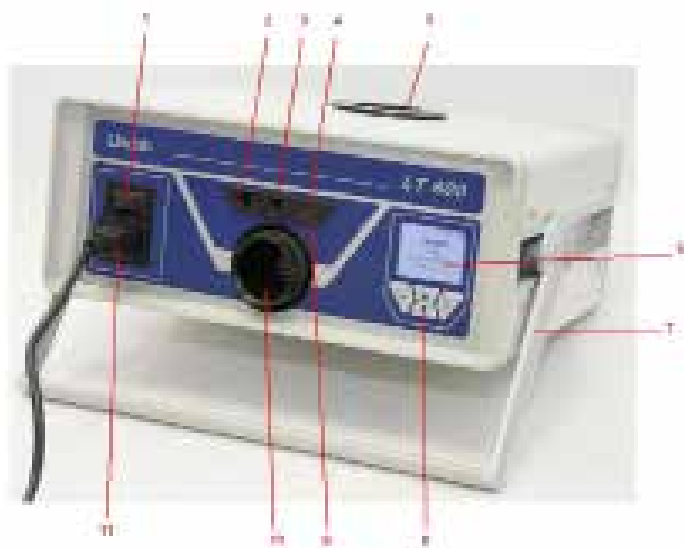
Bild 2: Manöverelement
