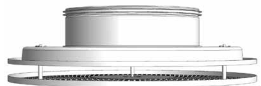
PCA
